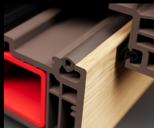
Výplň dolní kovací drážky
