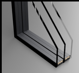
Izolační trojsklo U_g = 0,5 \text{ W(m}^2\text{K)} [ U_w = 0,73 \text{ W(m}^2\text{K)} ]
