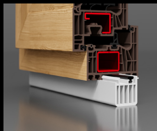
5-komorová podkladní lišta s těsněním
